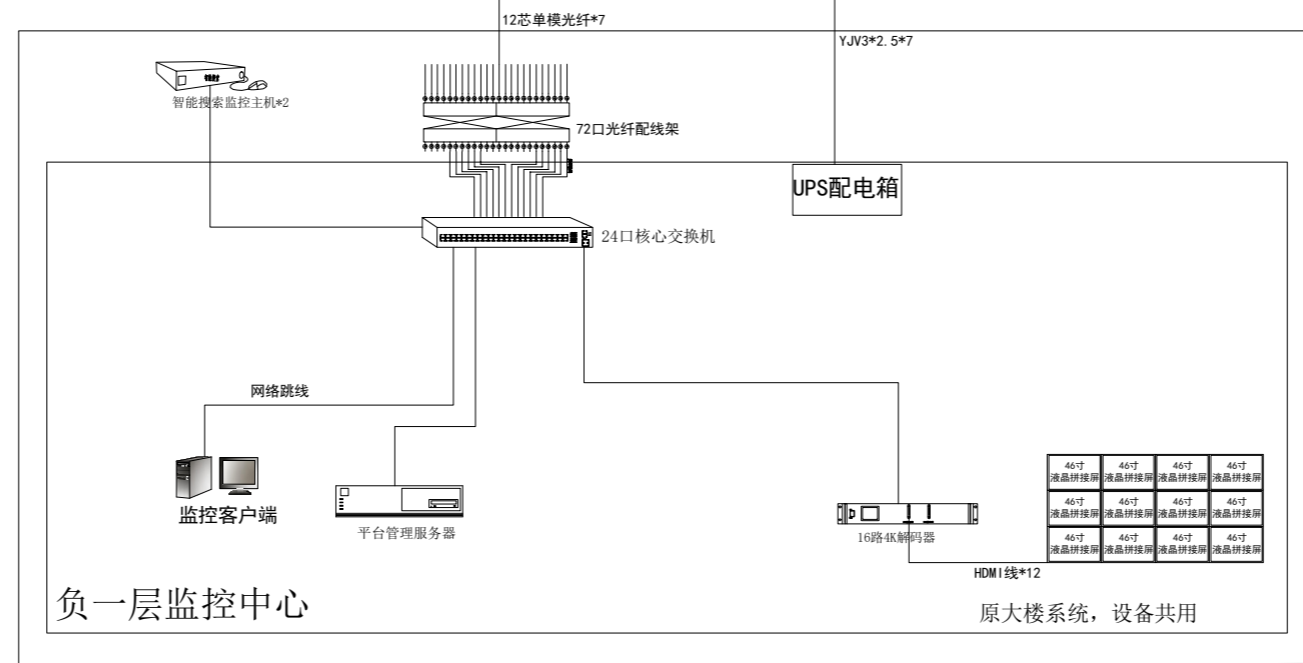
视频监控系统图
